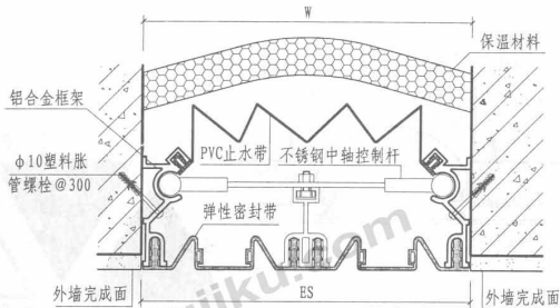
② 外墙（封缝型 WQP） （适合缝宽200~300）
