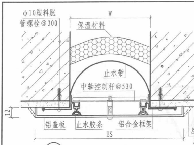
① 外墙（盖板型 WQPL）
