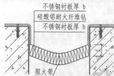
阻火带安装示意图
