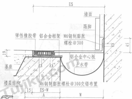
② a 楼、地面与墙面（嵌平式DJR）
