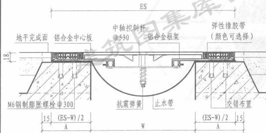
③ 楼、地面（抗震型DPRM）
