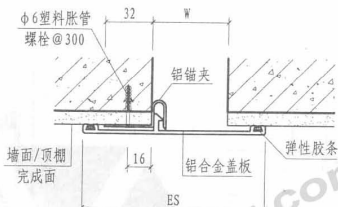
② 内墙/顶棚 (卡锁式 NPG)
