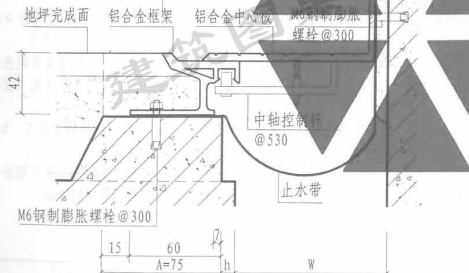
② b 楼、地面与墙面 (防滑型DJF)
