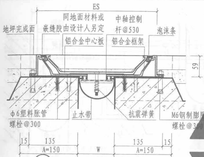
① 楼、地面 (抗震型DPS)
