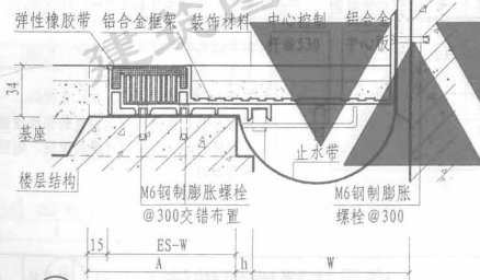
② b楼、地面与墙面（嵌平式DJRS）
