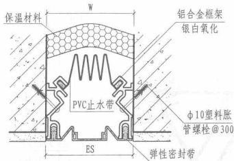
① 外墙（封缝型 WQP） （适合缝宽50~150）
