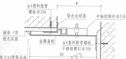
② 内墙/顶棚 (盖板型 NJL)
