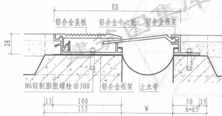
③ 楼、地面（卡锁式DPC）
