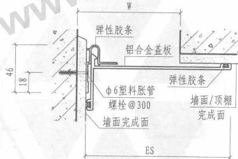
④ 内墙/顶棚 (卡锁式 NJG)
