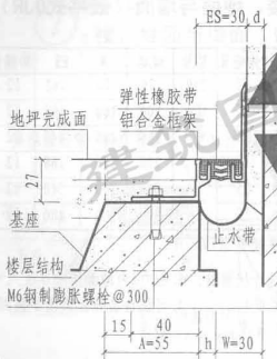
③ 楼、地面与墙面（嵌平式DJR-30）
