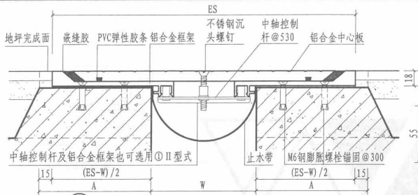
① a 楼、地面 (承重型DPZH)
