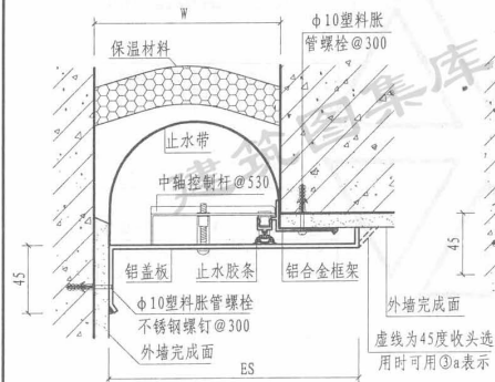
③ 外墙（盖板型 WQJL）
