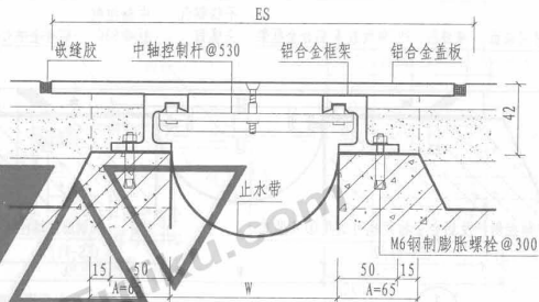
③ 楼、地面 (承重型DPZL)
