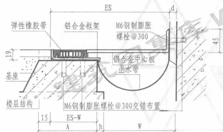
② b 楼、地面与墙面（嵌平式DJR）
