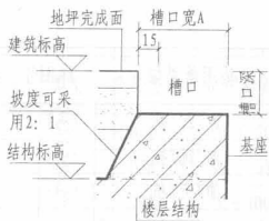
楼地面基座和槽口的三种形式:
