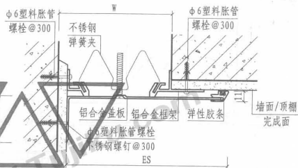
② 内墙/顶棚 (盖板型 NJC)
