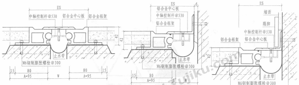
① 楼、地面（承重型DPZG）
