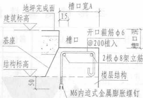
楼地面基座和槽口的三种形式:
