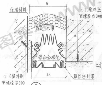
③ 外墙（封缝型 WQJ）
