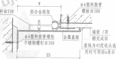
④ 内墙/顶棚 (盖板型 NJL-II)
