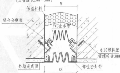
④ 外墙（封缝型 WQR）
