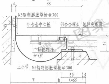
② b 楼、地面与墙面（盖板型DPL）
