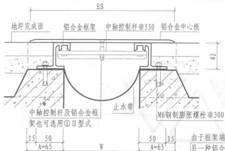
① a 楼、地面（盖板型DPL）
