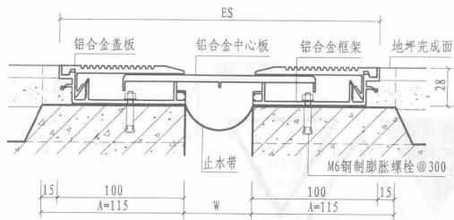
① 楼、地面（卡锁式DPK）
