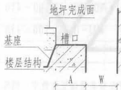
楼、地面与墙面 (2)
