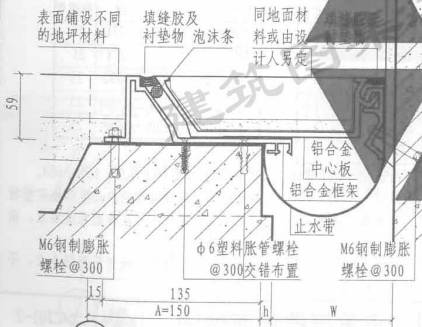
② 楼、地面与墙面 (抗震型DJS)
