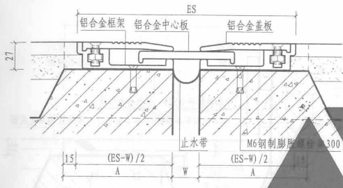
① 楼、地面 (承重型DPZL)
