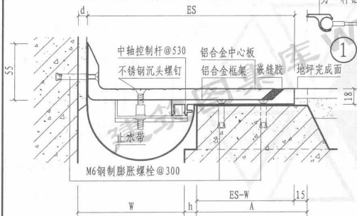
② b 楼、地面与墙面 (承重型DJZH)
