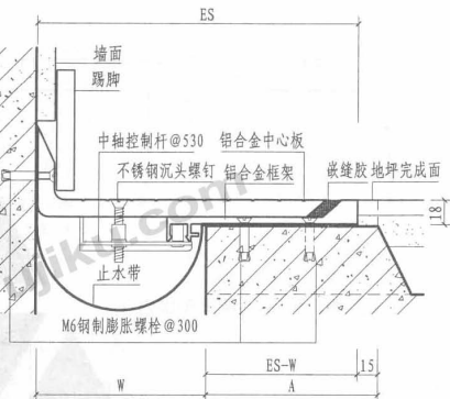
② a 楼、地面与墙面 (承重型DJZH)
