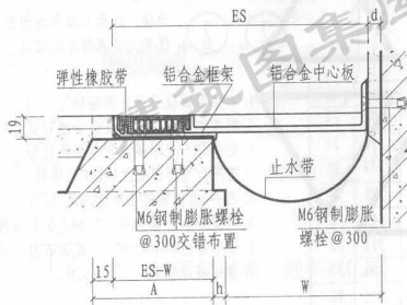
② b 楼、地面与墙面（嵌平式DJRSC）
