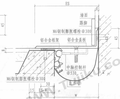
① b 楼、地面与墙面（盖板型DJLH）
