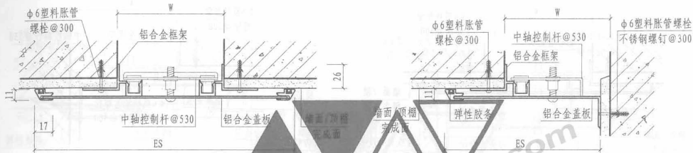
① 内墙/顶棚 (盖板型 NPH)
