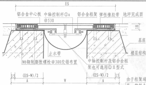
① a 楼、地面（嵌平式DPR）
