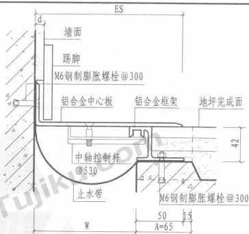
② a 楼、地面与墙面（盖板型DPL）
