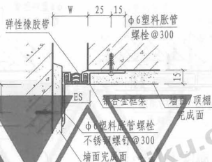
② 内墙/顶棚 (嵌平式 NJR)
