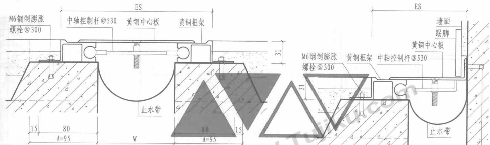
① 楼、地面 (盖板型DPPT)
