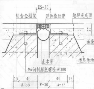
① 楼、地面（嵌平式DPR-30）
