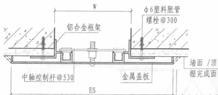
① 内墙/顶棚 (盖板型 NPL)
