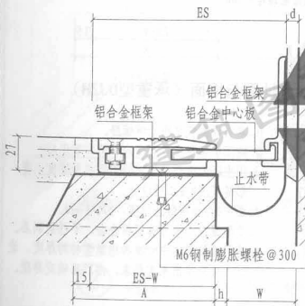
② 楼、地面与墙面 (承重型DJZL)
