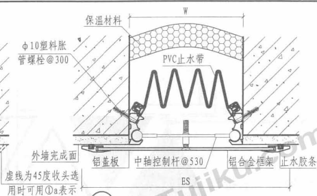
② 外墙（盖板型 WQPH）
