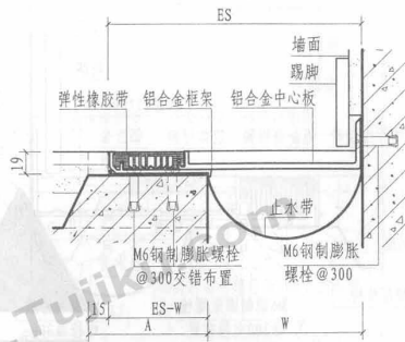
② a 楼、地面与墙面（嵌平式DJRSC）
