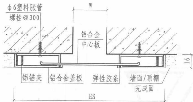
① 内墙/顶棚 (卡锁式 NPK)
