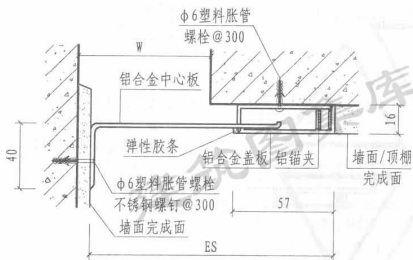
③ 内墙/顶棚 (卡锁式 NJK)
