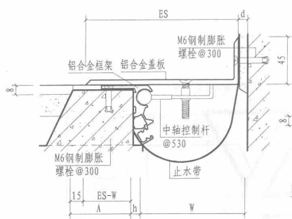
① a 楼、地面与墙面（盖板型DJLH）
