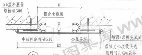
③ 内墙/顶棚 (盖板型 NPL-II)
