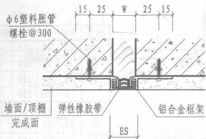
① 内墙/顶棚 (嵌平式 NPR)
