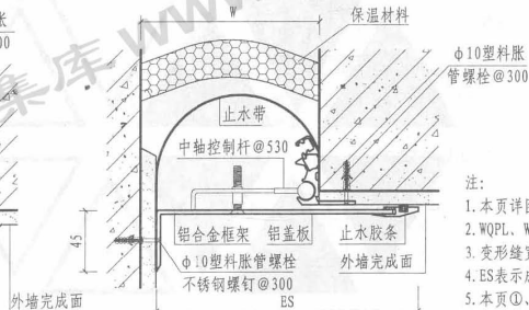
④ 外墙（盖板型 WQJH）
