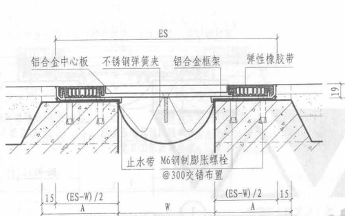
① 楼、地面（双列嵌平式DPRSC）
