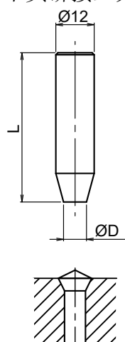
平头铆接工具
